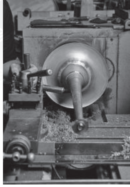
円盤状の板を高速で回転させながら 力を加えてベルの形に絞っていく
